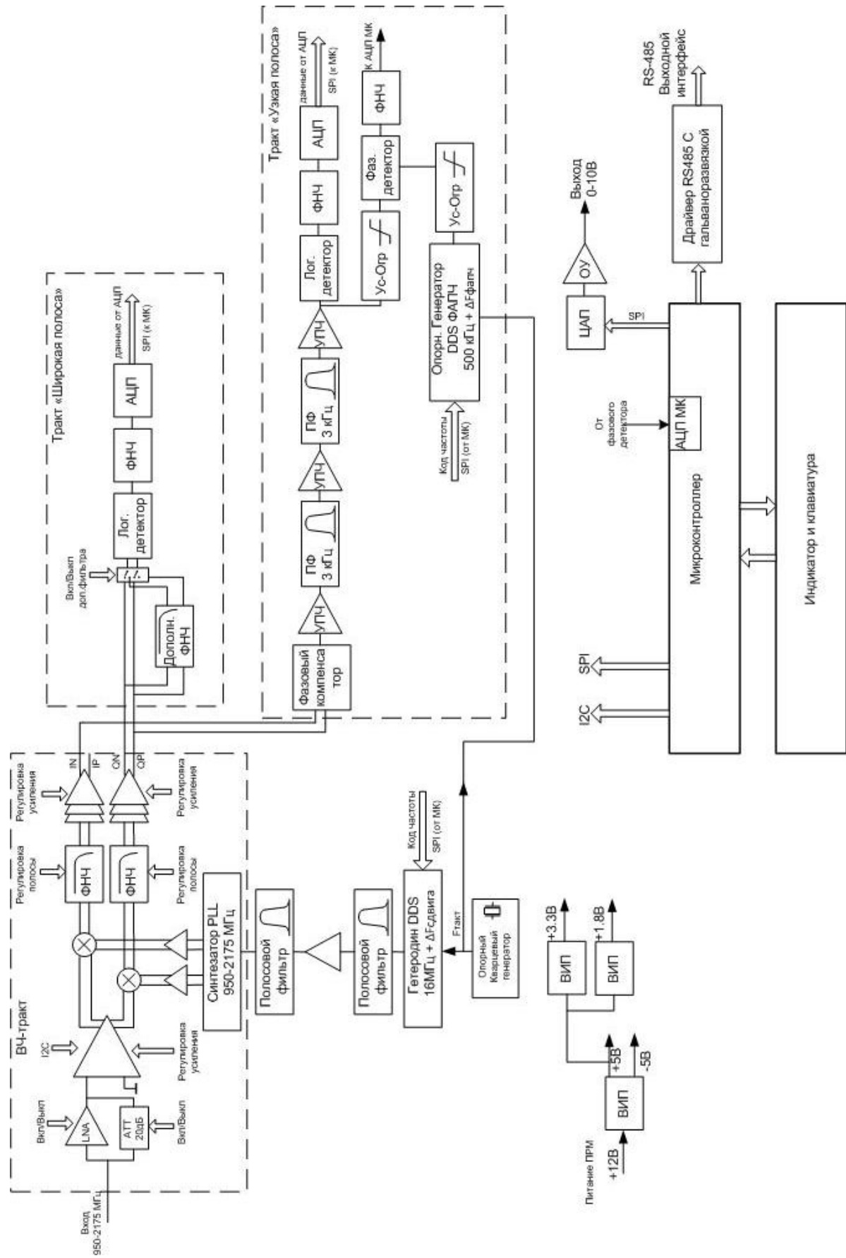
Рисунок 1.2.2.2 - Функциональная схема приемника сигнала наведения ПСН
