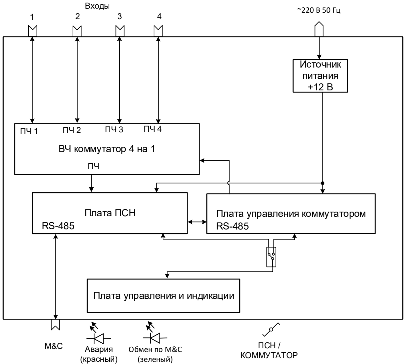
Рисунок 1.2.1 – функциональная схема блока ПСН
